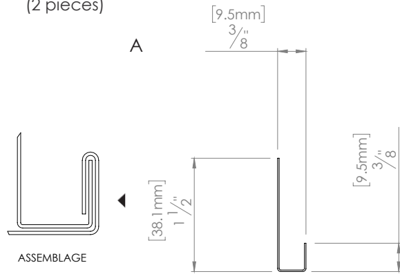
No. M03D (NW & NWM) J Trim à palette variable (2 pièces)
