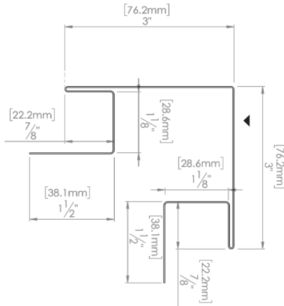
No. M21A (SPC1.1) Coin extérieur avec J intégrés
