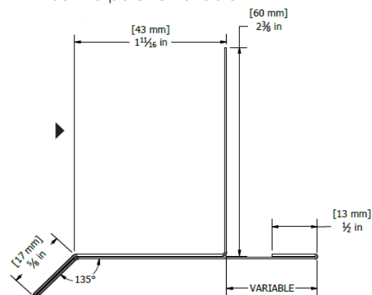
No. M56J (SPC1.2, SPC1.3) Solon à palette variable
