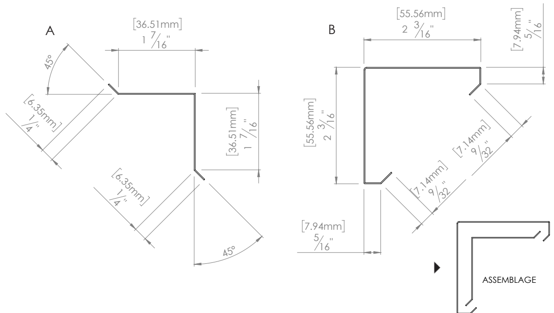
No. M20C ((HWP, HW, HWB & MS 14) Coin extérieur (2 pièces)
