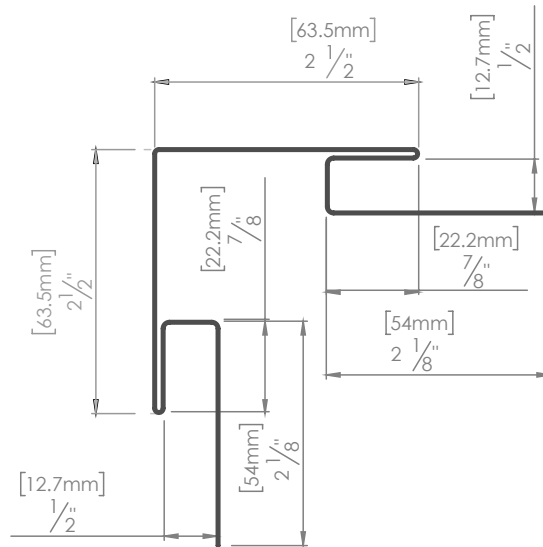
No. M20D (NW & NWM) Coin extérieur avec J intégrés
