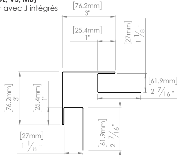
No. M20G (POL, VS, MB) Coin extérieur (2 pièces)
