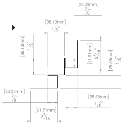
No. M22IA (SPC1.1) Coin intérieur avec J intégrés
