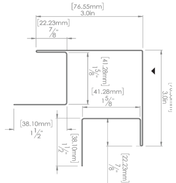
No. M21B (SPC1.2, SPC1.3) Coin extérieur avec J intégrés
