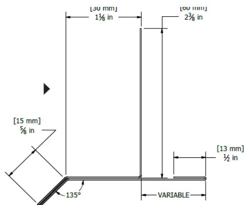
No. M56I (SPC1.1) Solon à palette variable
