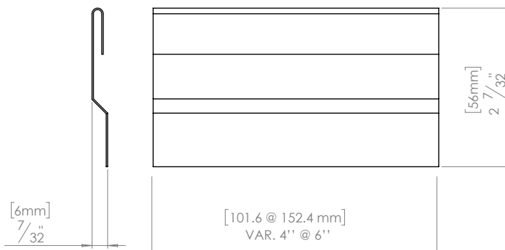
No. ABRA2 (HW) Braquette de soutènement arrière
