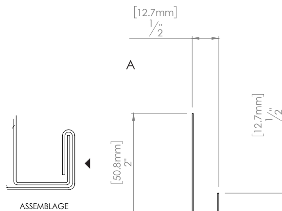
No. M03D (NW & NWM) J Trim à palette variable (2 pièces)
