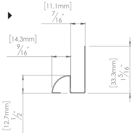
No. M22C (HWP, HW, HWB & MS 14) Moulure en QJ ou coin intérieur
