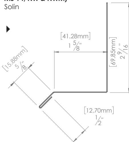
No. M56CD (HWP, HW, HWB, MS 14, NW & NWM) Solin à palette variable
