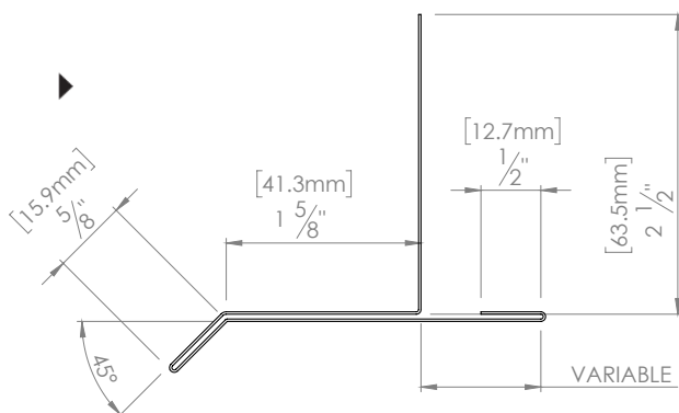
No. M56CD (HWP, HW, HWB, MS 14, NW & NWM) Solin à palette variable
