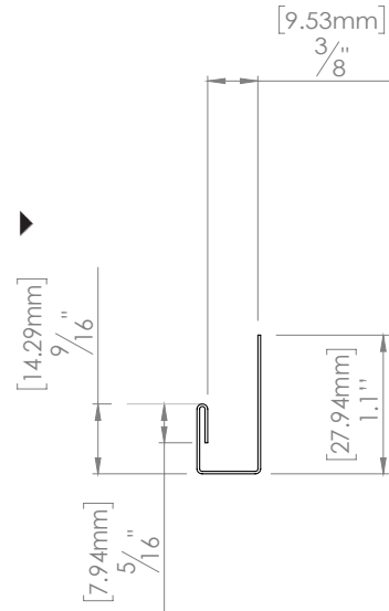
No. M03C ((HWP, HW, HWB & MS 14) J Trim à palette variable (2 pièces)
